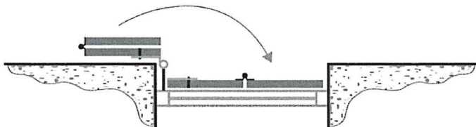
Anschlagsart 3 Doppelflügel einseitig liegend = 2 Flügel
