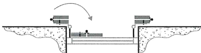
Anschlagsart 5 Doppelflügel beidseitig = 4 Flügel
