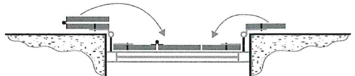
Anschlagsart 4 doppelflügelig + einflügelig = 3 Flügel
